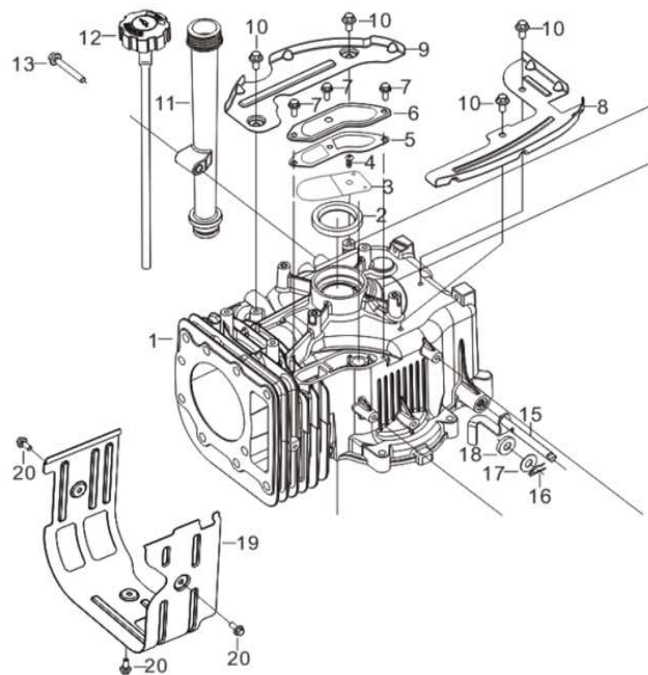
FIG.1 CRANKCASE.
