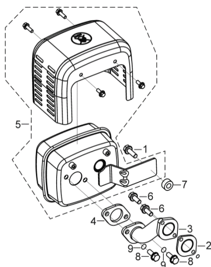
FIG.11 MUFFLER
